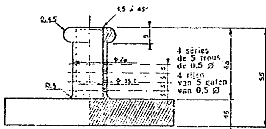
CORPS/CILINDER — Echelle/Schaal : 1 : 2 — Bronze/Bronz
