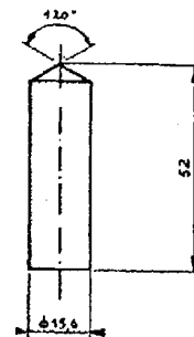
PISTON/ZUIGER — Echelle/Schaal : 1 : 2 — Bronze/Bronz
