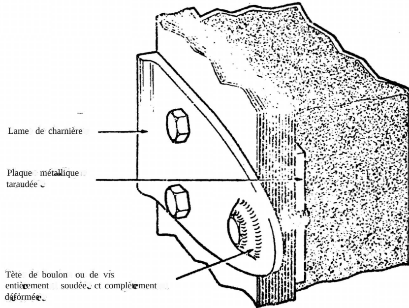
Charnière
